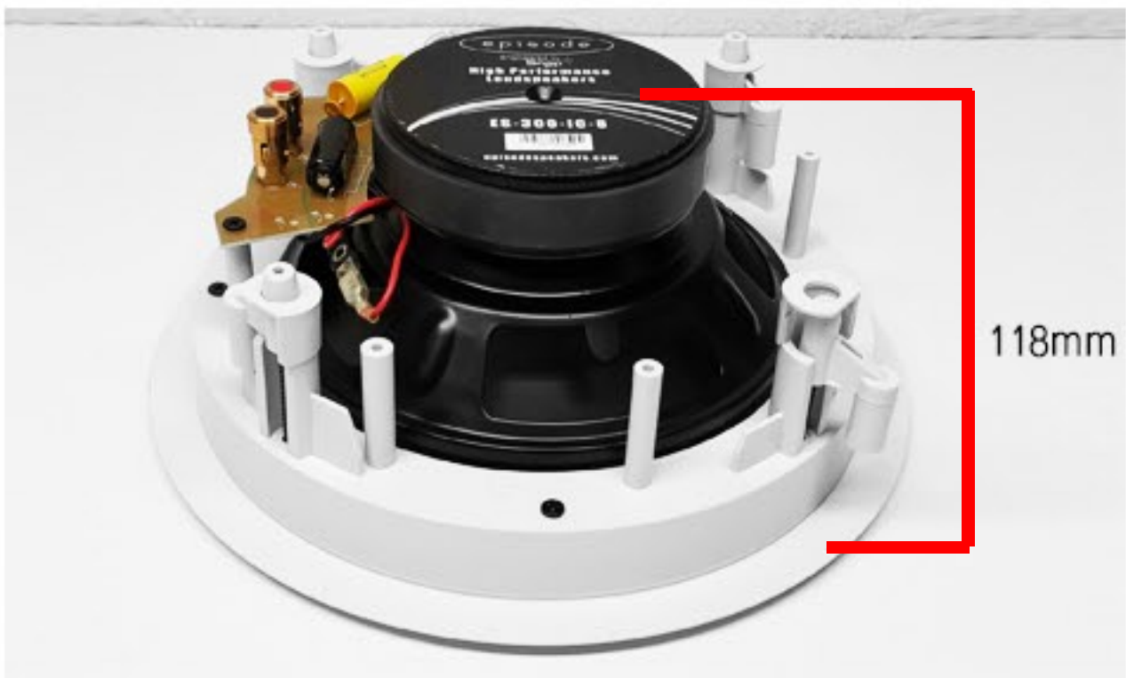
安裝深度
